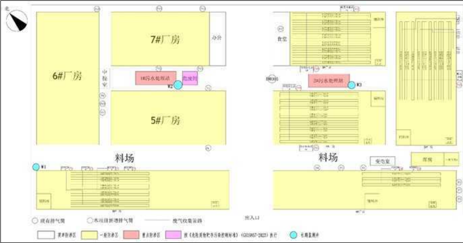
图 8.5-1 本项目污染防治分区及地下水跟踪监测井示意图
