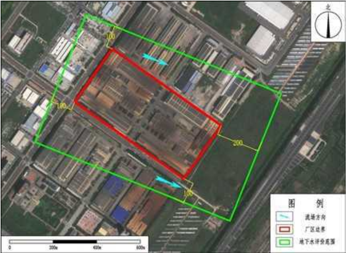
图 1.7-2 地下水调查评价区范围
