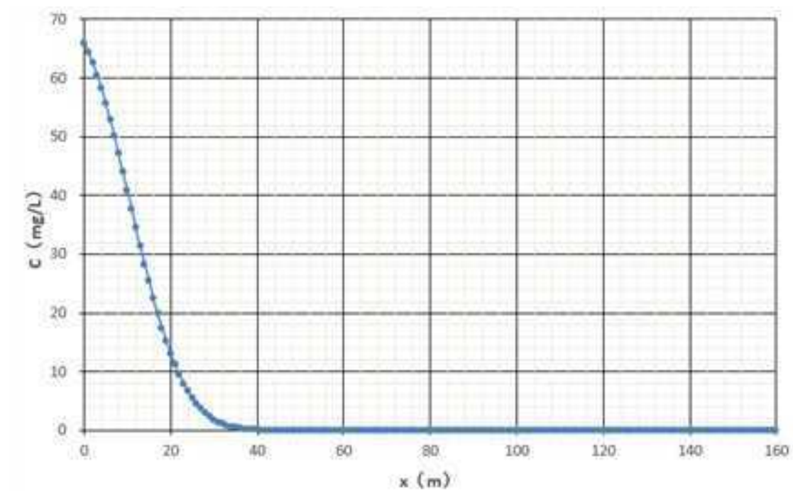
图 5.6-7 10 年时泄漏点下游地下水中铁浓度-距离 (C-x) 关系
