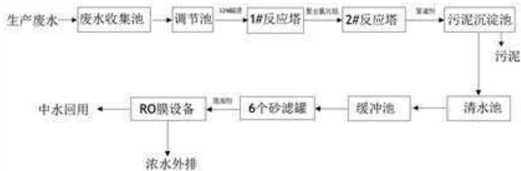
图 3.8-1 污水处理站处理工艺流程图
